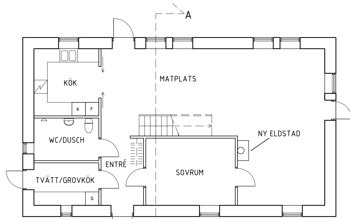
PLAN BOTTENVÅNING
