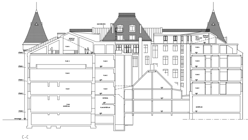
Sektions- och fasadritning som visar påbyggnad mot gården och balustrad på taknocken.
